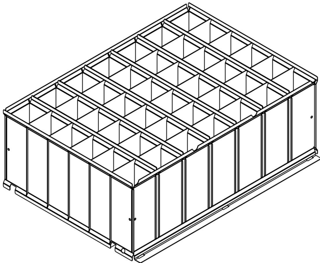
Комплект разделителей Н-220
