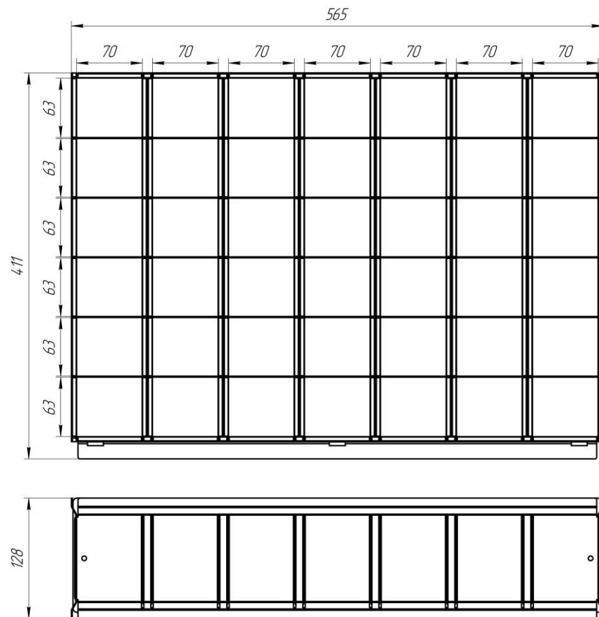
4.4. Габаритные размеры комплекта разделителей Н-220.
