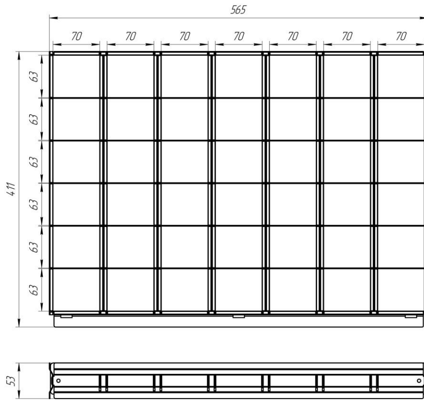
4.3. Габаритные размеры комплекта разделителей Н-145.
